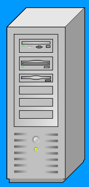
SQL 2000 Server
